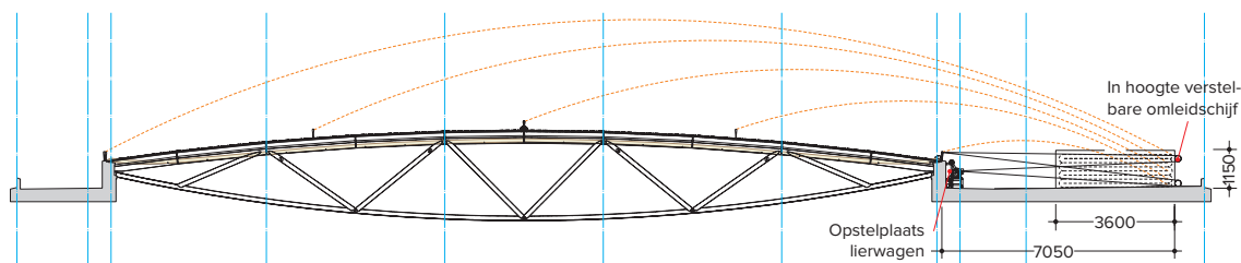
DEMONTAGE LUCHTKUSSENDAK
